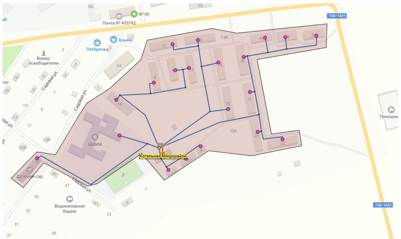
Рисунок 4 – Зона действия источников теплоснабжения р.п. Старотимошкино (Котельная "Микрорайон" (р.п. Старотимошкино, ул. Микрорайон, 1))
