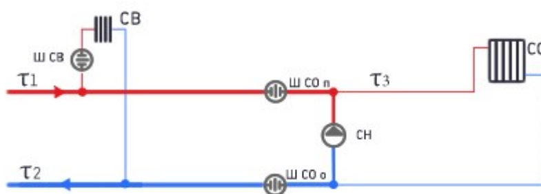
Рисунок 3 – Схема подключения потребителей к двухтрубной тепловой сети (при наличии внутридомовой системы отопления), СО – система отопления, СН – насос системы отопления, СВ – система вентиляции
