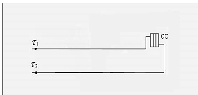
Рисунок 1 - Схема подключения потребителей к двухтрубной тепловой сети (при наличии внутридомовой системы отопления), зависимое присоединение, без смешения
