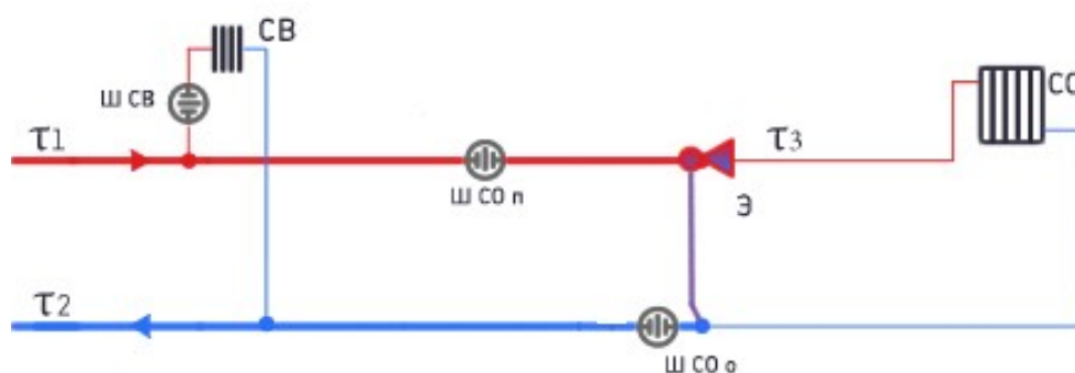
Рисунок 2 – Схема подключения потребителей к двухтрубной тепловой сети (при наличии внутридомовой системы отопления), в качестве регулятора температуры используется элеватор (СО – система отопления, Э – элеватор, СВ – система вентиляции)
